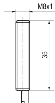
Габаритный чертеж
